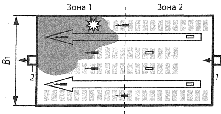
б) Очаг пожара в зоне 1
