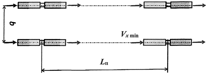
а) Соосная установка струйных вентиляторов
