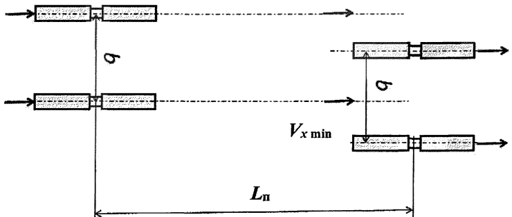
б) Параллельная установка струйных вентиляторов
