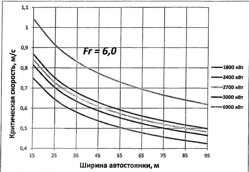
Рисунок Е.1 – График зависимости V_{кр} от ширины автостоянки B при различных значениях конвективной мощности пожара Q_{кв} , при числе Фруда Fr = 6,0
