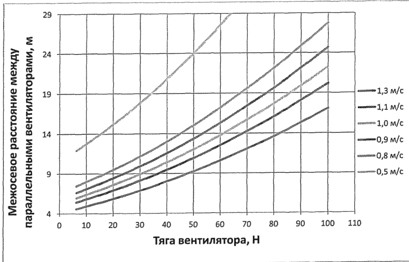
Рисунок И.2 – График зависимости межосевого расстояния b от расчетной реактивной тяги вентилятора F_p при различных значениях
