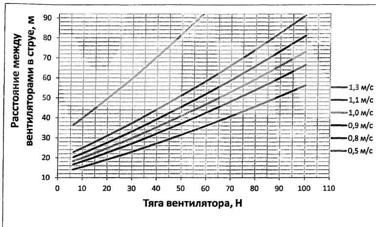
Рисунок И.1 – График зависимости расстояния L_p (в струе) от расчетной реактивной тяги F_p вентилятора при различных значениях
