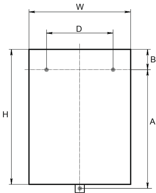
Габариты настенных шкафов IP54.
