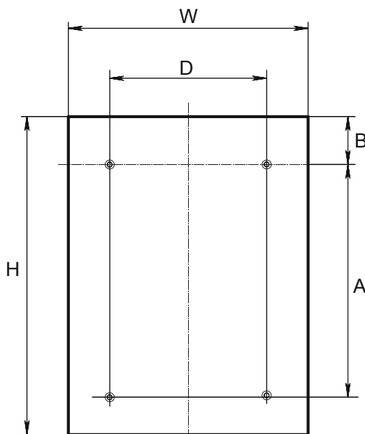
Габариты настенных шкафов IP31.
